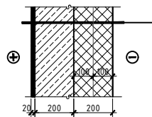
Гадна ханын бүтэц M1:20
