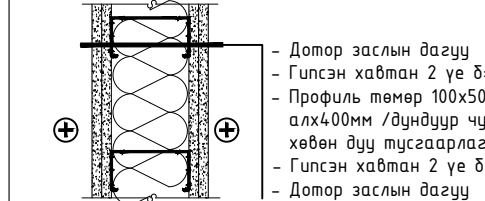
Дотор ханы бүтэц /Гүлсэн хана/ M1:10
