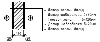
Дотор ханын бүтэц /Тоосгон хана/ M1:20
