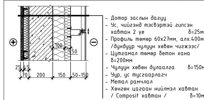
Гадна ханы бүтэц M1:20
